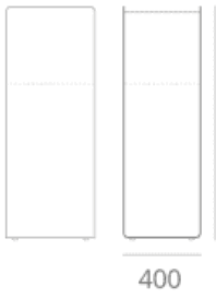
CREPE_H
