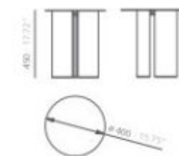
BEDSIDE TABLE
