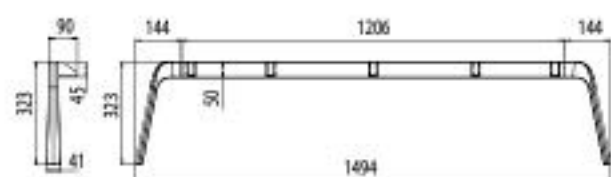
ELI_FDE3 Kit fianco doppio esterno con viti Double outer side kit with screws Kit mit doppelter Außenseite und Schrauben
