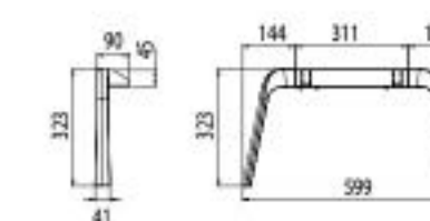
ELI_FSE3 Kit fianco singolo esterno con viti Single outer side kit with screws Kit einzelne Außenseite und Schrauben
